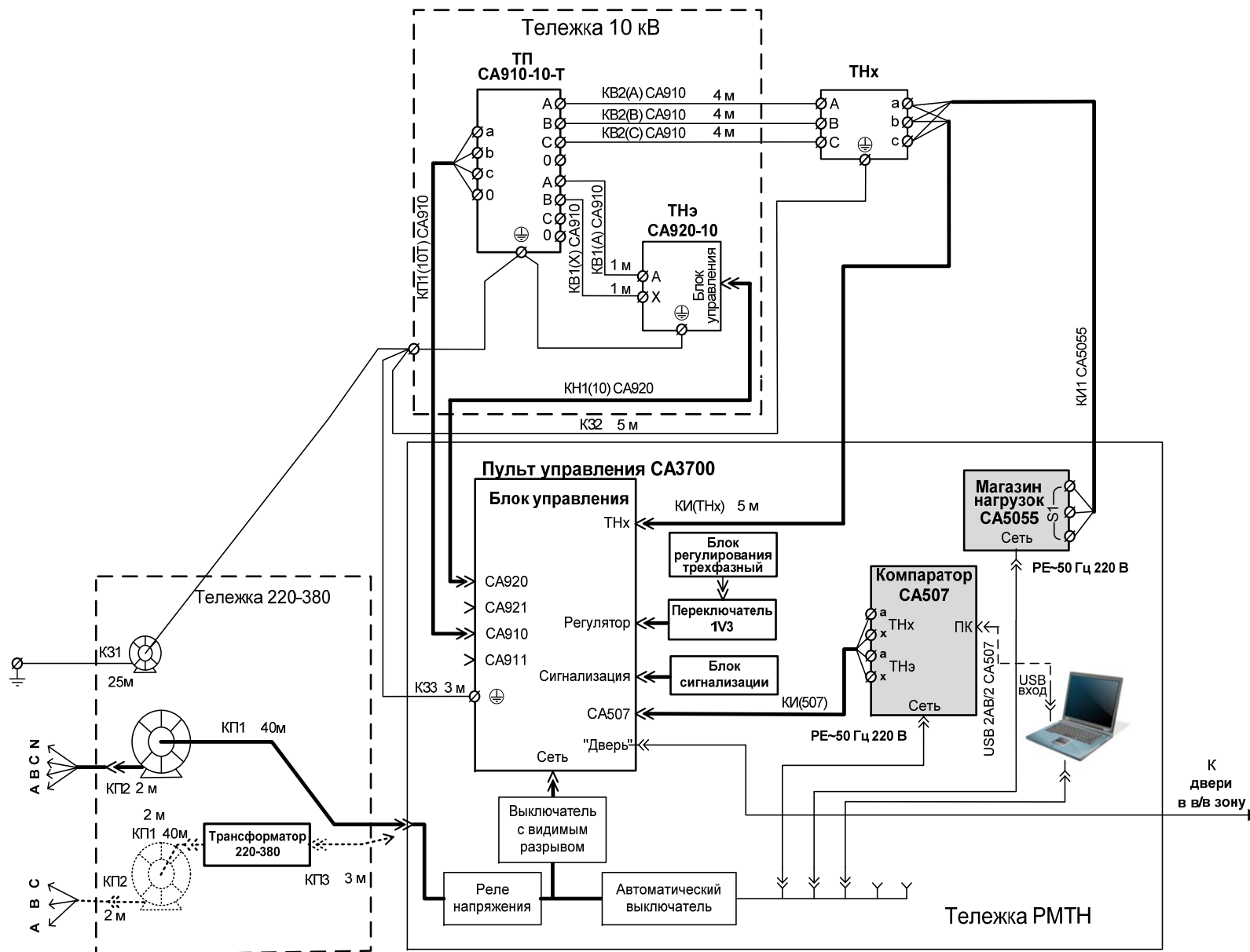
Схема поверки трехфазного ТН
