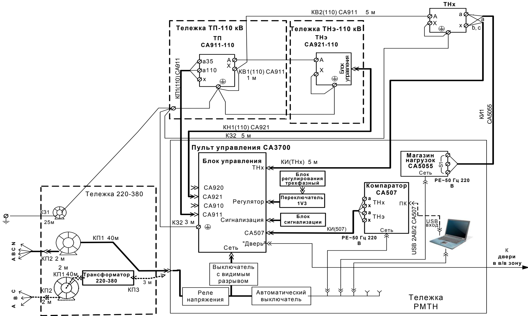
Схема поверки однофазного ТН
