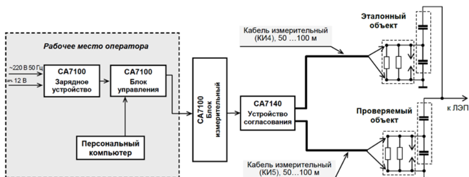
Рис. Схема подключения Устройства CA7140 и Моста CA7100 к объекту измерения
