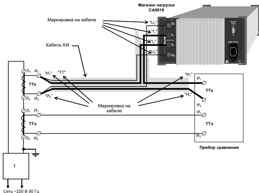
1 – источник тока ТТх – поверяемый или калибруемый трансформатор тока; ТТэ – эталонный трансформатор тока
