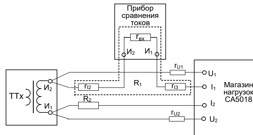
R_2, r_a, r_b, r_{U1}, r_{U2} – сопротивления проводов подключения; r_{вх} – входное сопротивление прибора сравнения
