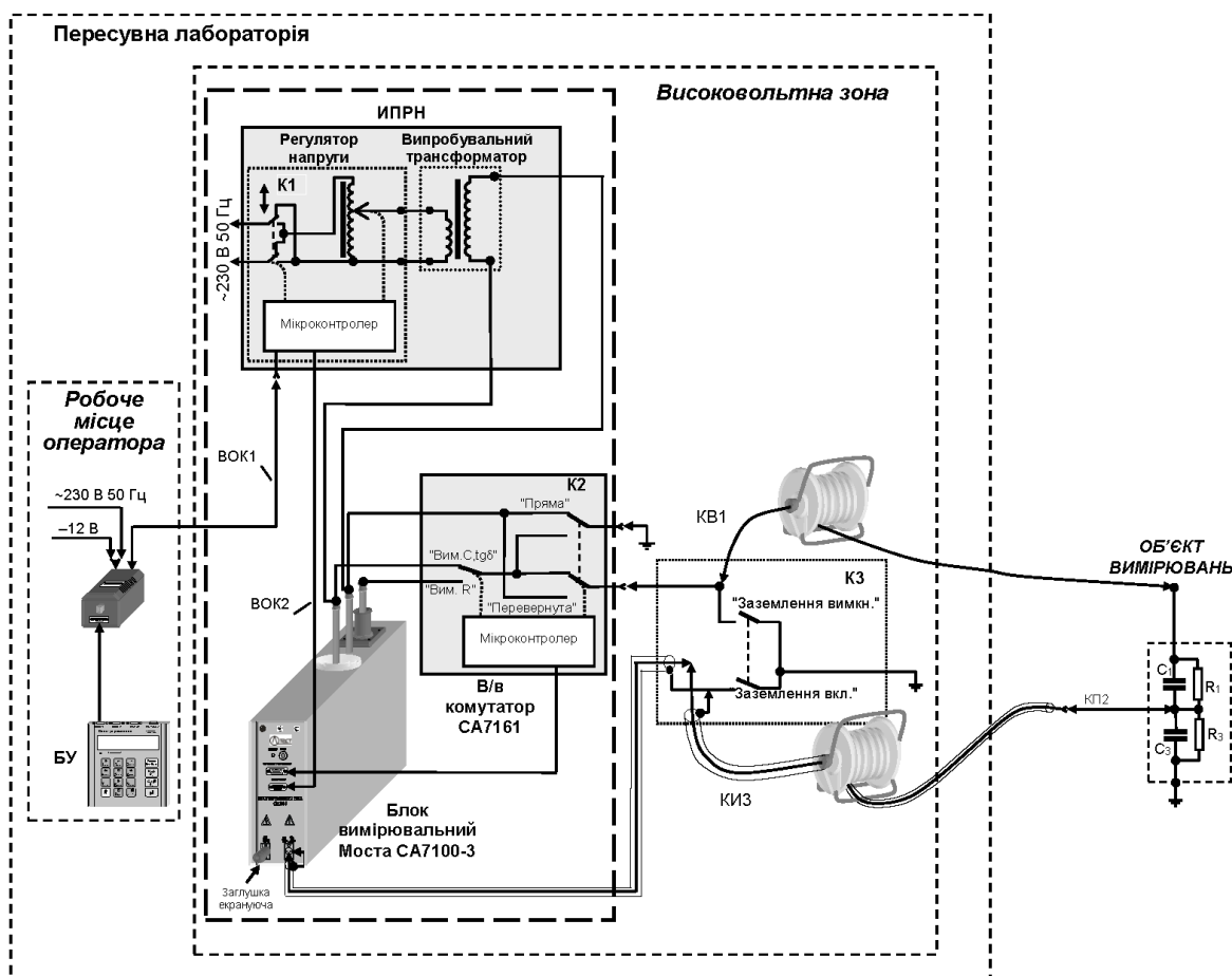
Рис. Схема підключення Комплекту CA7100-2K
