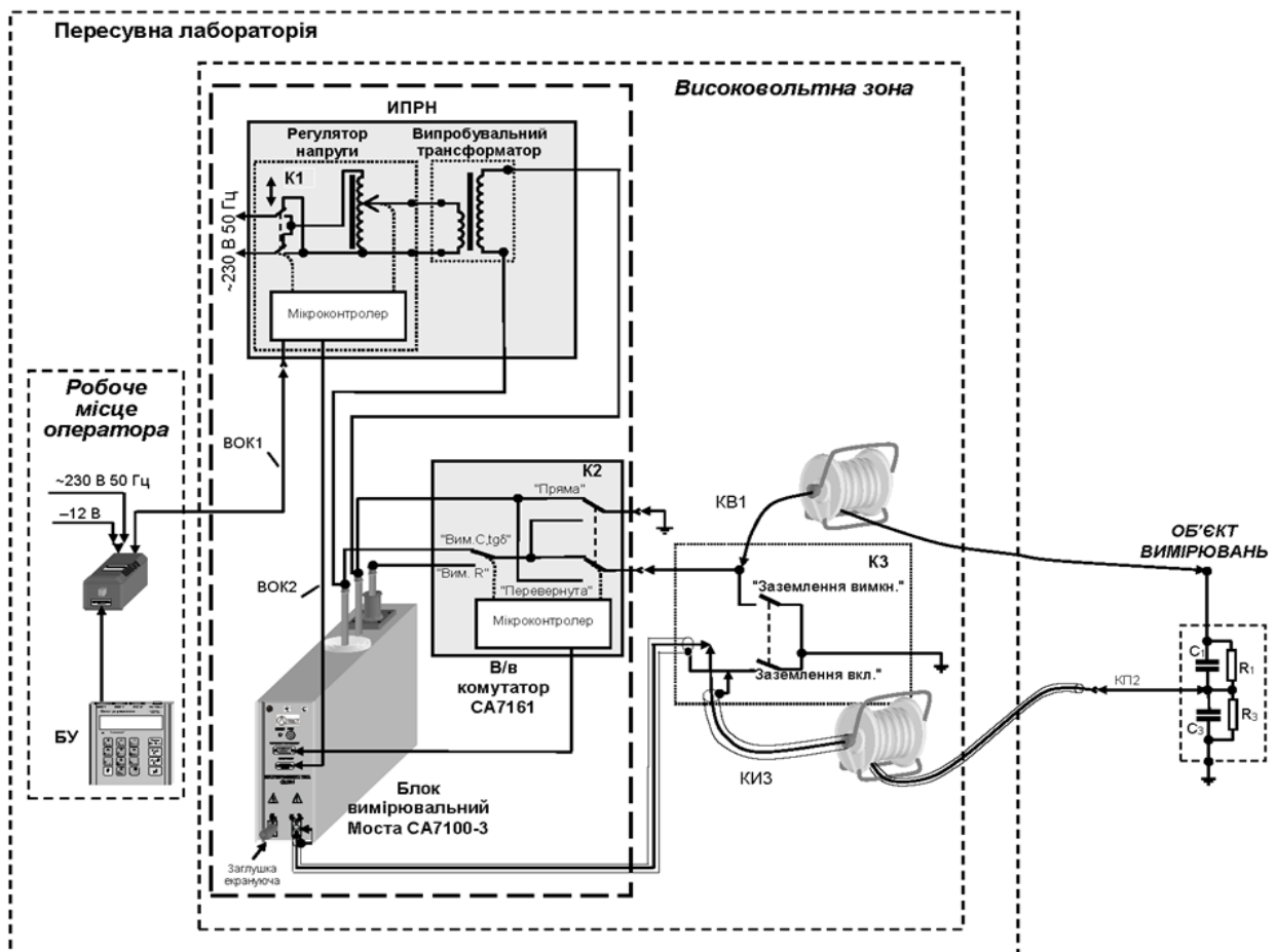
Рис. Схема підключення Комплекта CA7100-3КП
