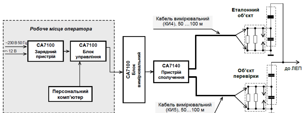
Рис. Схема підключення Пристрою СА7140 і Моста СА7100 до об'єкта перевірки
